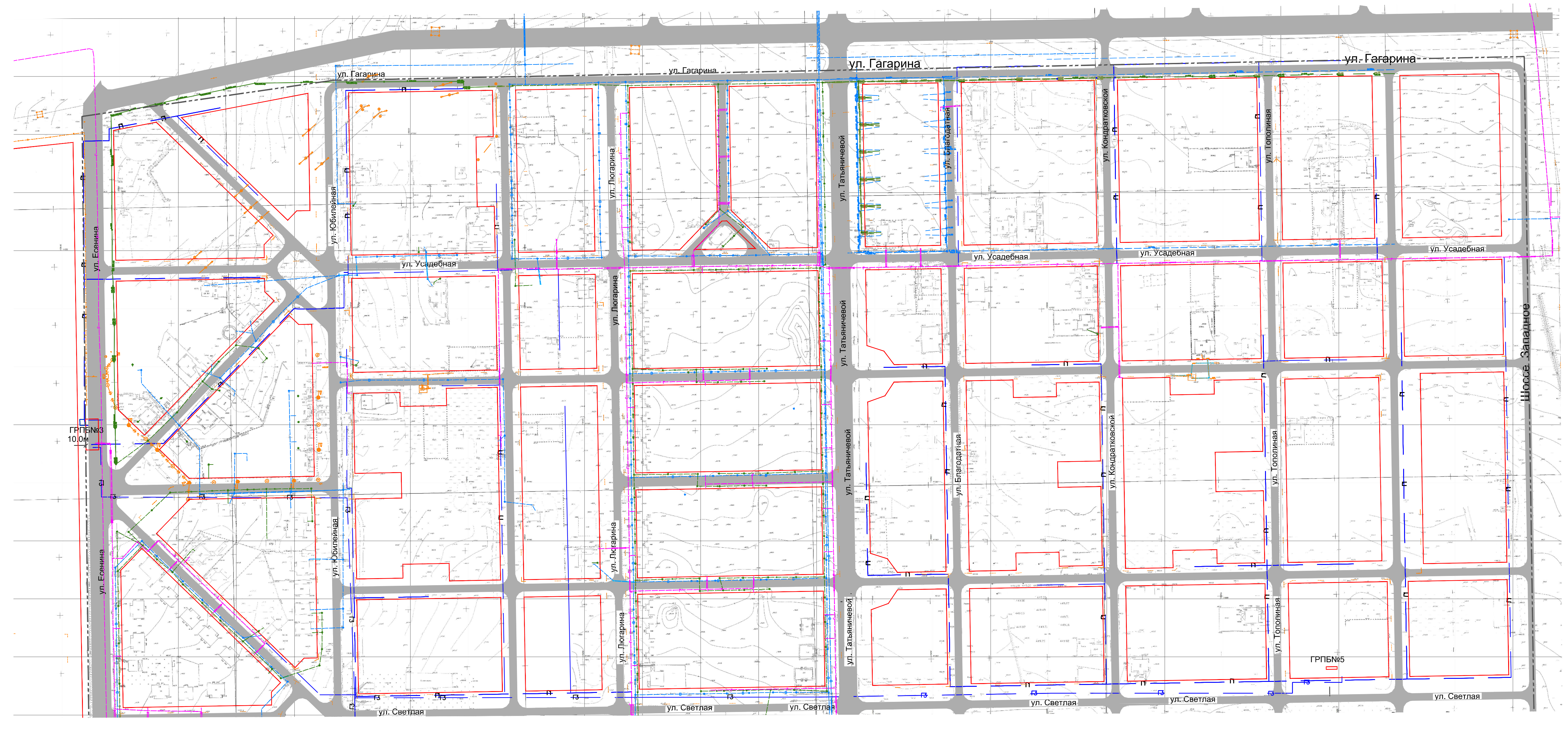
План красных линий. Схема планировки территории. Основной чертеж (1:2000)
