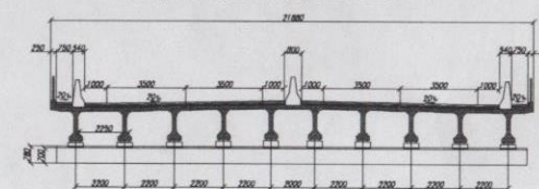
Поперечный разрез пролетного строения
