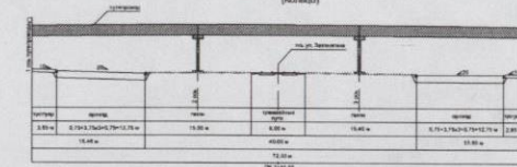
Поперечный конструктивный профиль ул. Завенягина ПК 2+00.00 М1:200
