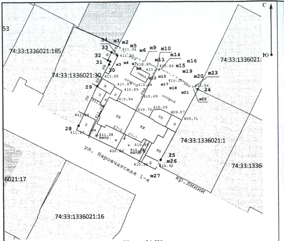
Масштаб 1:500
