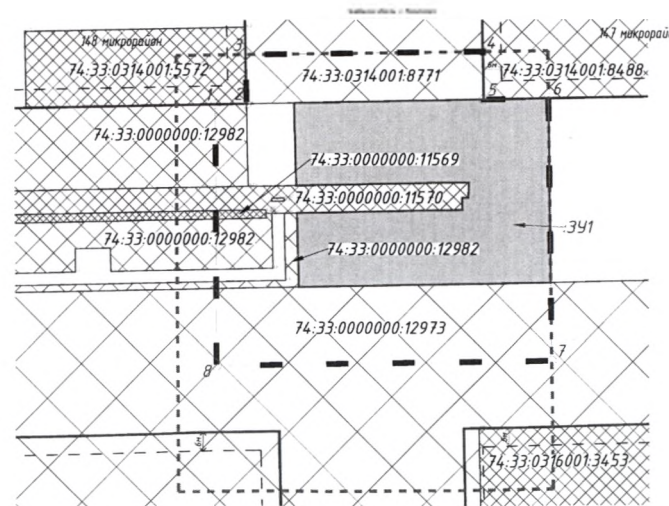
Чертеж межевания территории
