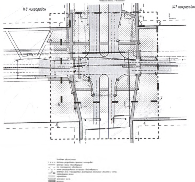
Чертеж границ зон планируемого размещения линейного объекта
