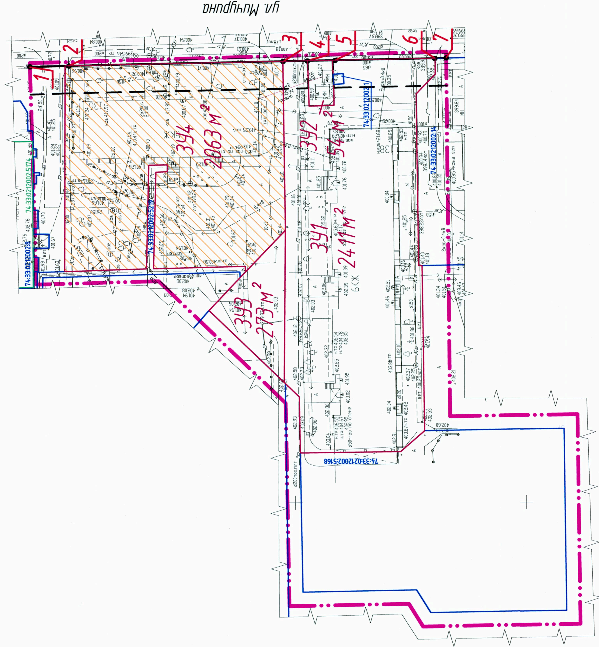
Чертеж межевания территории. 3 вариант 2 этап. М 1:500
