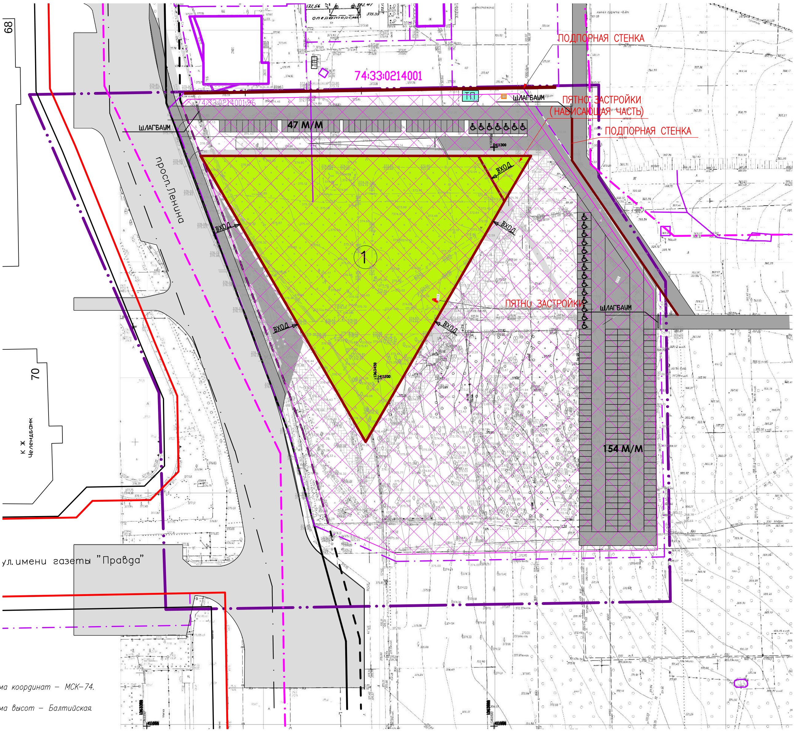
Чертеж планировки территории (М 1:1000)
