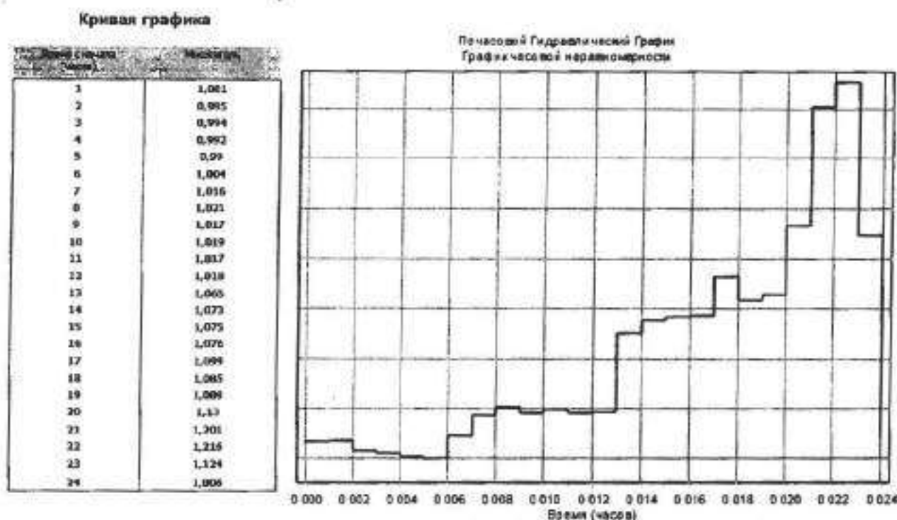
Рисунок 60 - График суточной неравномерности
