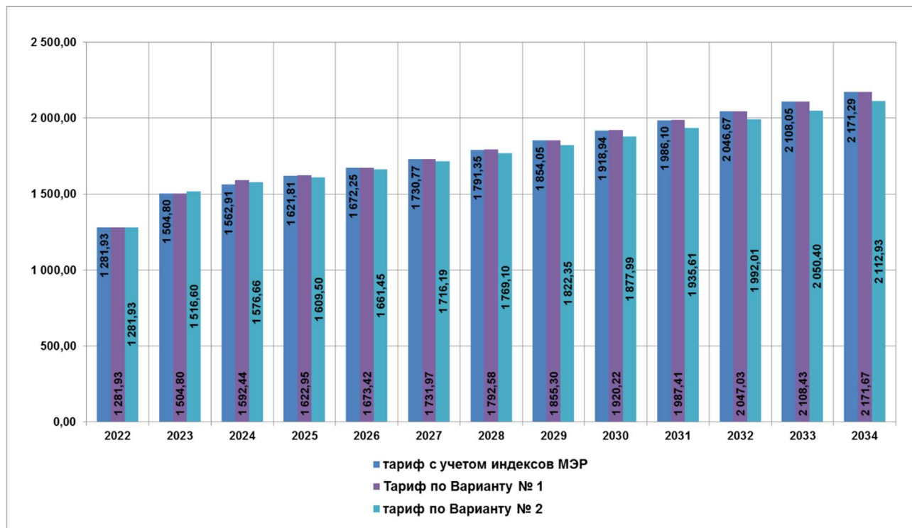
Рисунок 3. Прогнозируемый уровень тарифа конечного потребителя в зоне действия ЕТО № 1 по двум Вариантам развития системы теплоснабжения
