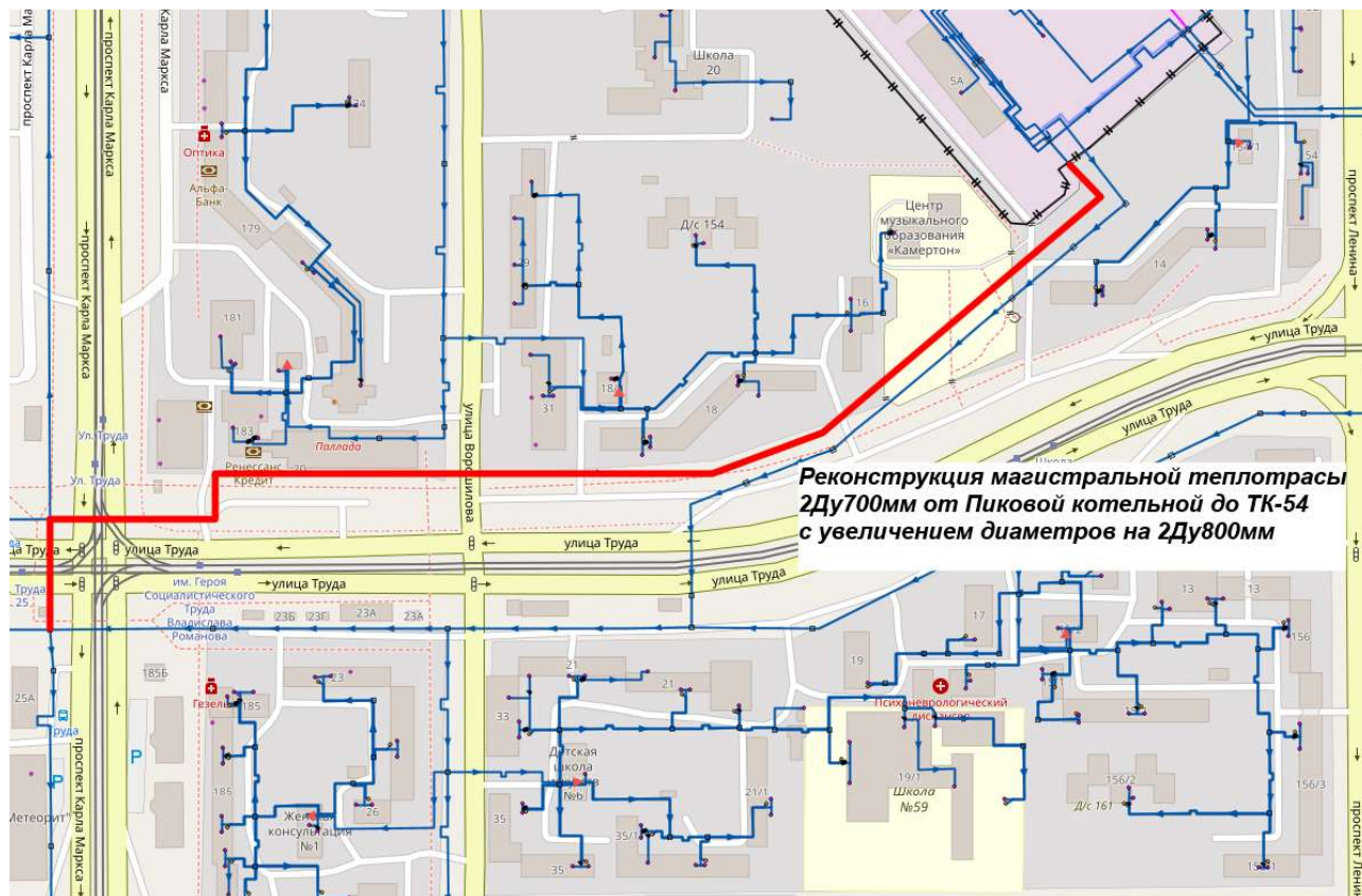
Рисунок 1. Схема реконструкции участка теплотрассы от ТП-12 до ТК-155 (отмечена красным цветом)
