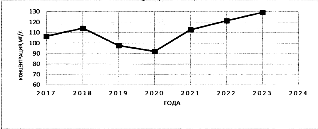
Рисунок 34 - Изменение концентрации взвешенных веществ в сточных водах, поступающих на Левобережные очистные сооружения
