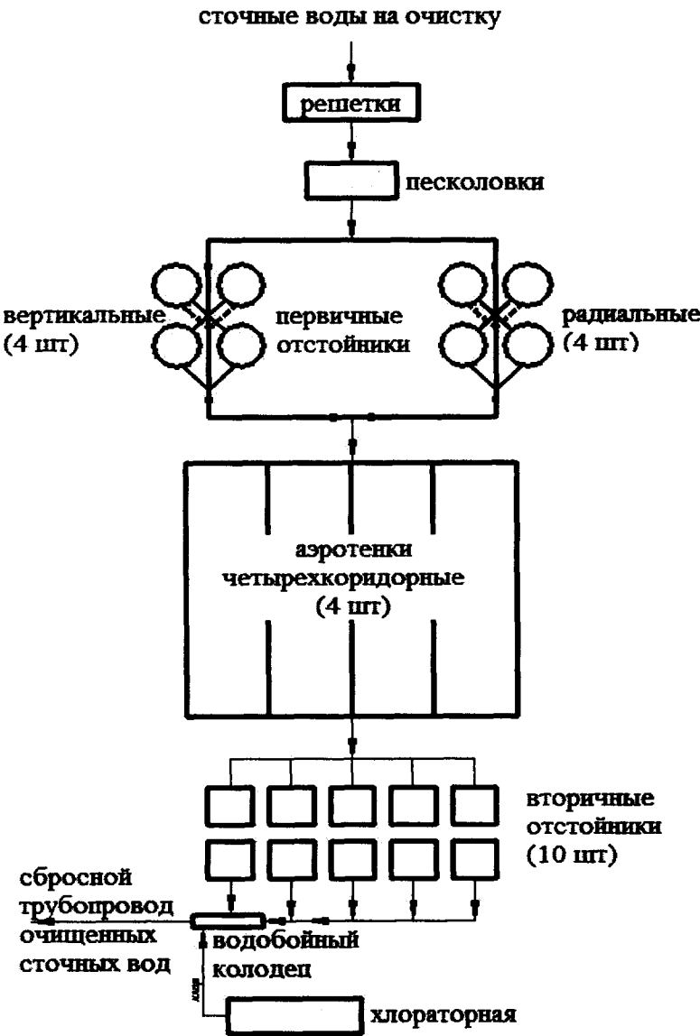
Рисунок 31 – Принципиальная технологическая схема Левобережных очистных сооружений канализации
