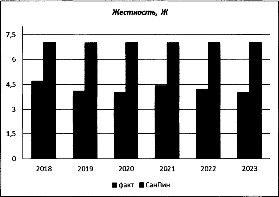
Рисунок 3 – Колебание жесткости воды Мало-Кизильского водозабора
