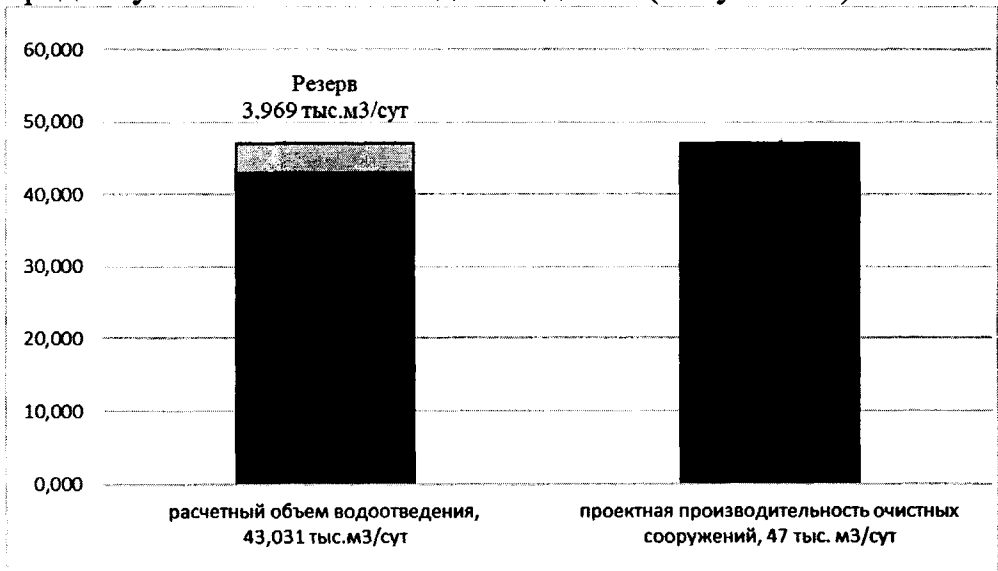
Рисунок 54 - Анализ резервов и дефицитов производственной мощности левобережных очистных сооружений на расчетный срок
