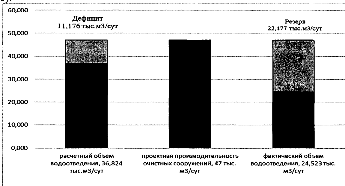
Рисунок 51 - Анализ резервов и дефицитов производственной мощности левобережных очистных сооружений за 2023 г.
