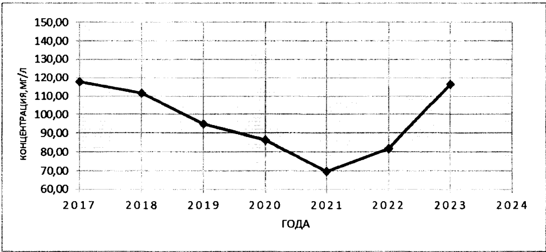
Рисунок 35 - Изменение концентрации загрязнений по БПК в сточных водах, поступающих на Левобережные очистные сооружения
