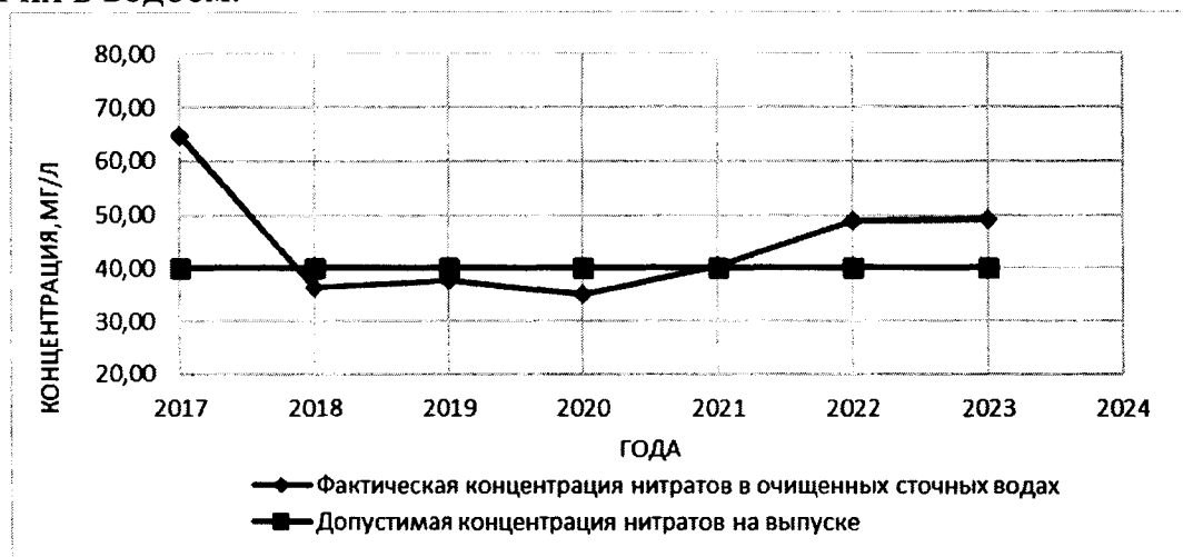
Рисунок 42 - Изменение концентрации нитратов в очищенных сточных водах на Левобережных очистных сооружениях
