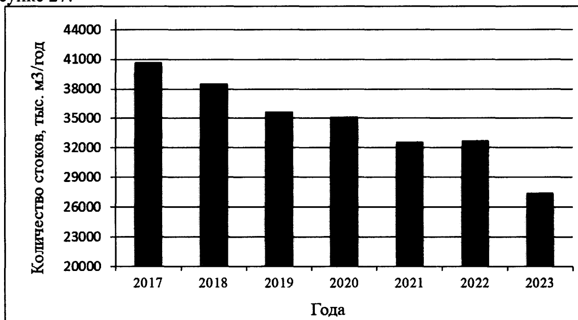
Рисунок 27 - Изменение годовых объемов сточных вод, поступивших на правобережные очистные сооружения в период с 2017 по 2023 гг.
