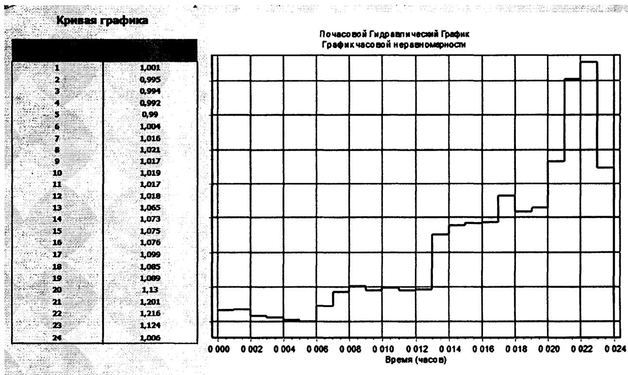
Рисунок 60 – График суточной неравномерности
