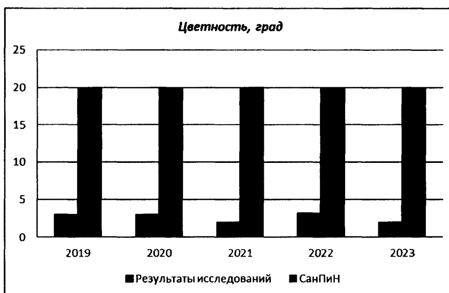
Рисунок 8 – Колебание цветности воды Янгельского водозабора
