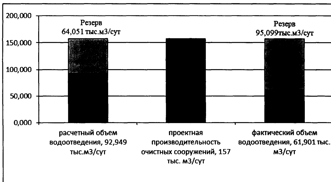
Рисунок 52 - Анализ резервов и дефицитов производственной мощности правобережных очистных сооружений за 2023 г.
