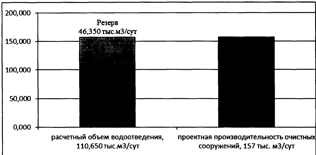
Рисунок 55 - Анализ резервов и дефицитов производственной мощности правобережных очистных сооружений на расчетный срок
