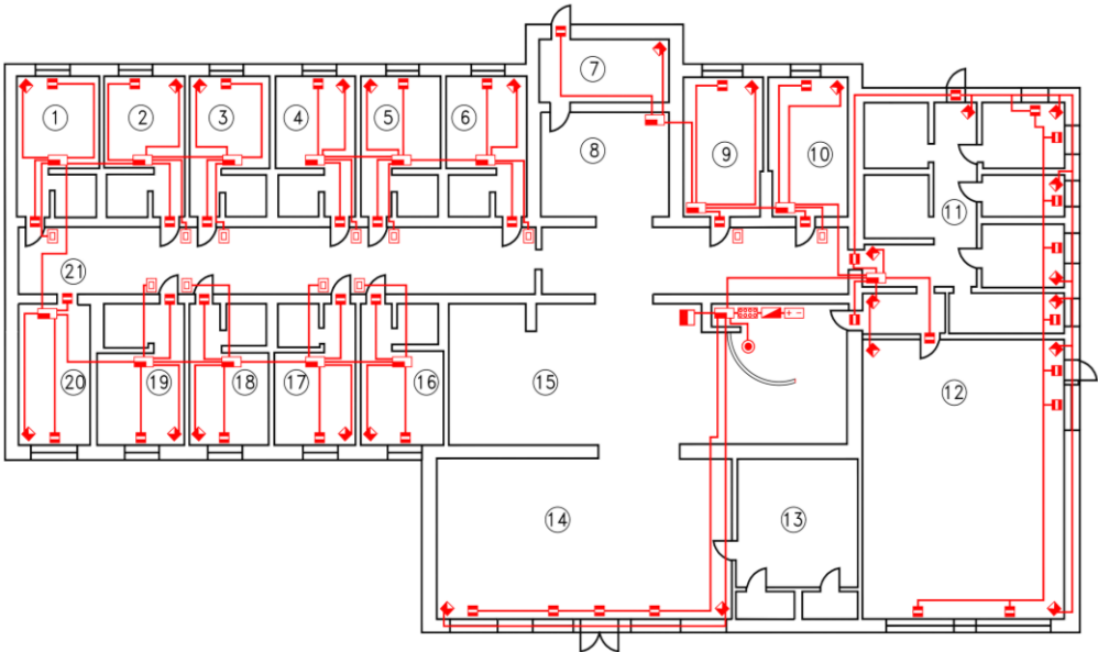
Экспликация помещений
